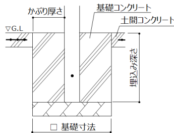
②土間コンクリート考慮基礎
