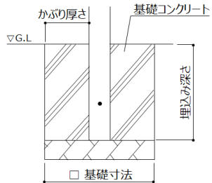
①独立基礎
