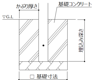
①独立基礎
