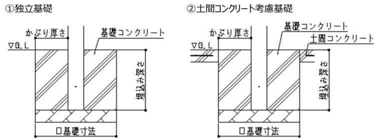
図1.基礎仕様
