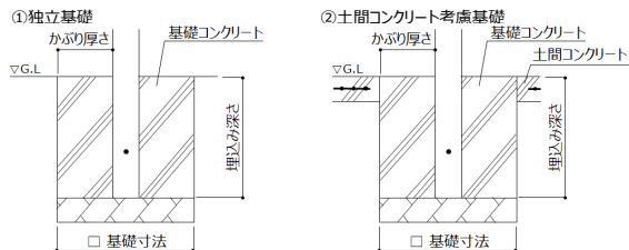
図1. 基礎仕様
