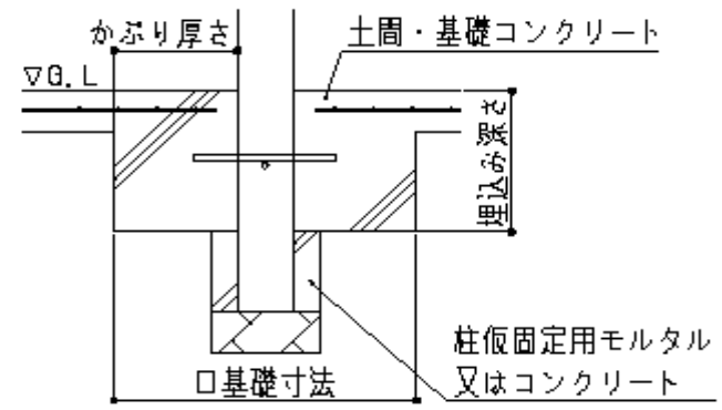
③土間コンクリート一体基礎
