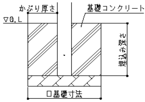
①独立基礎
