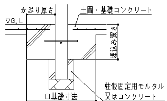
③土間コンクリート一体基礎
