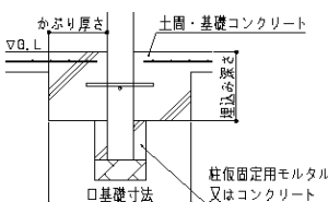
③土間コンクリート一体基礎
