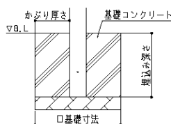
①独立基礎
