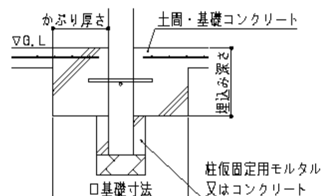
③土間コンクリート一体基礎
