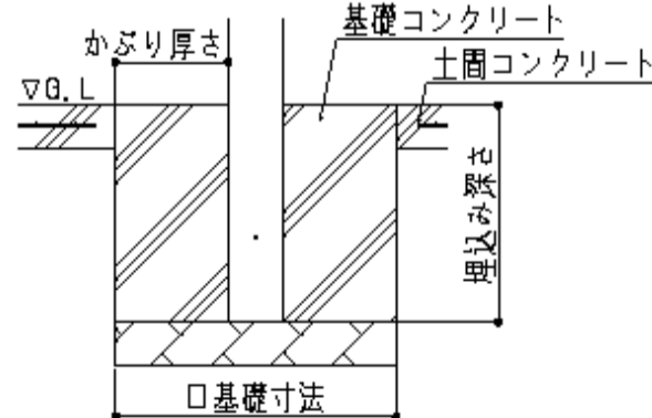
図1.基礎仕様
