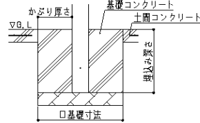
図1.基礎仕様
