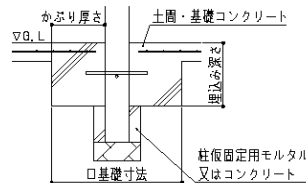
③土間コンクリート一体基礎
