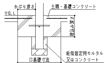
③土間コンクリート一体基礎
