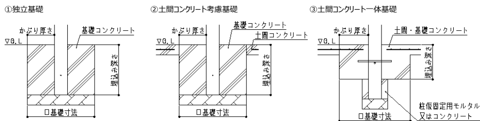
図1.基礎仕様
