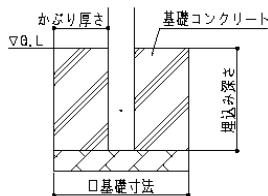
①独立基礎
