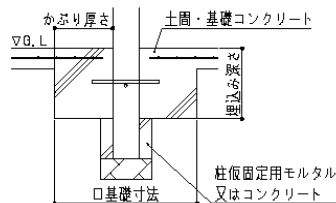
③土間コンクリート一体基礎
