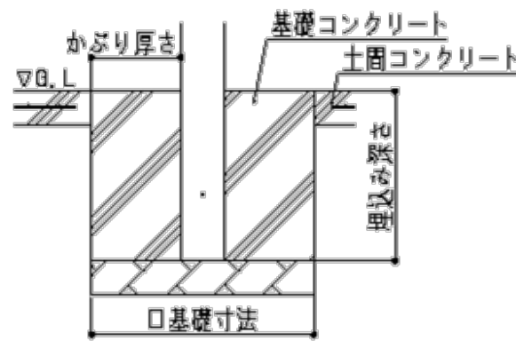
②土間コンクリート考慮基礎
