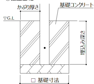
①独立基礎
