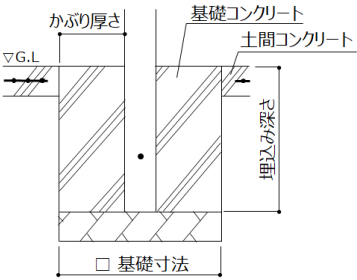
②土間コンクリート考慮基礎
