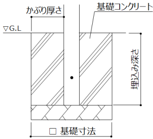
①独立基礎
