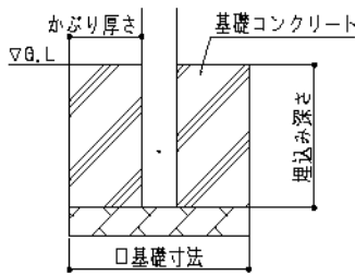
①独立基礎
