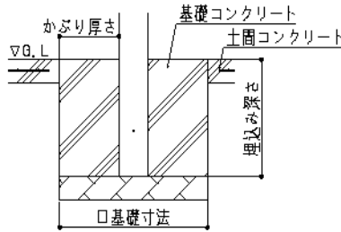
②土間コンクリート考慮基礎
