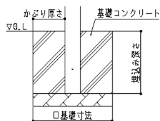
①独立基礎
