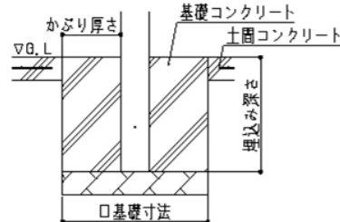
②土間コンクリート考慮基礎
