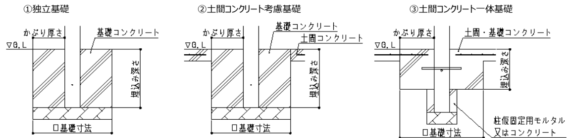
図1.基礎仕様
