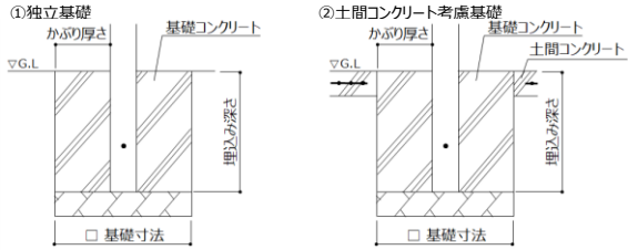
図1. 基礎仕様
