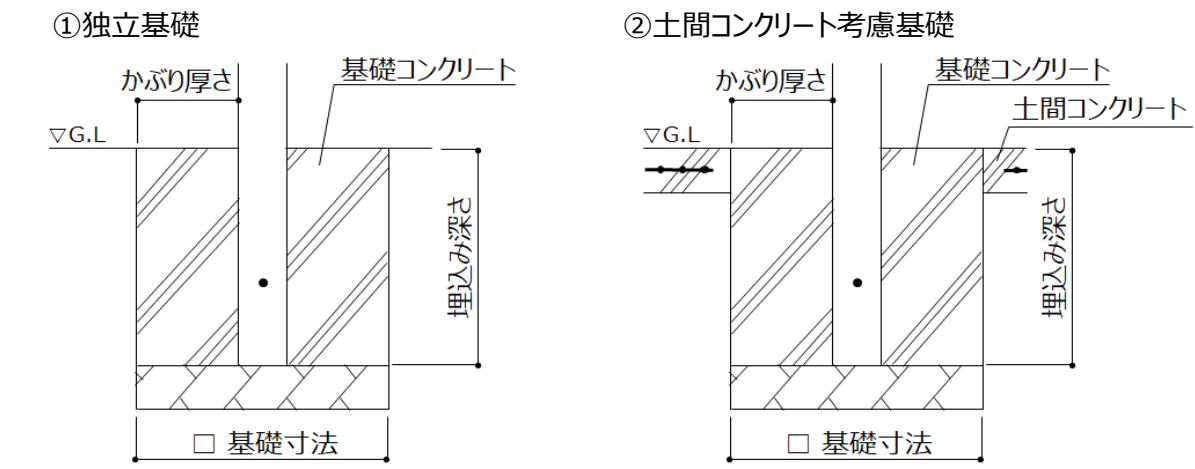
図1. 基礎仕様
