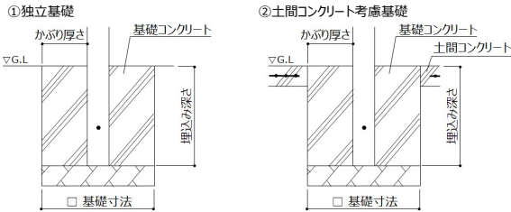
図1. 基礎仕様
