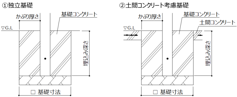
図1. 基礎仕様
