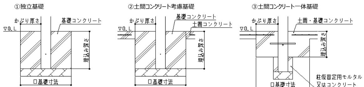
図1.基礎仕様
