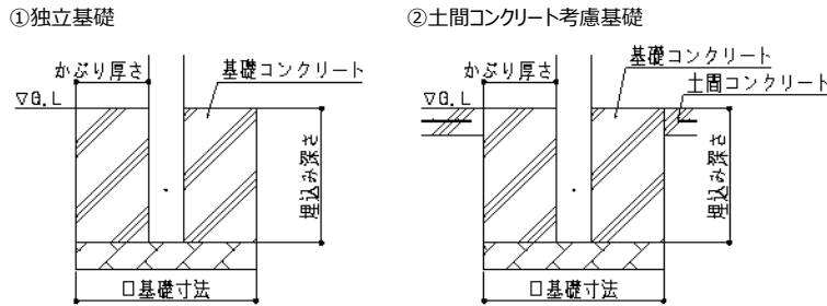
図1.基礎仕様
