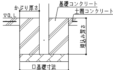
図1.基礎仕様
