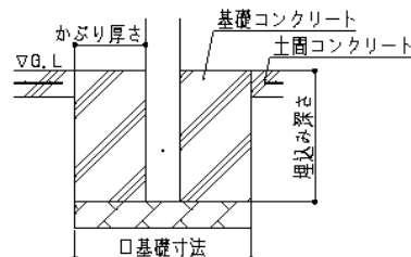
②土間コンクリート考慮基礎
