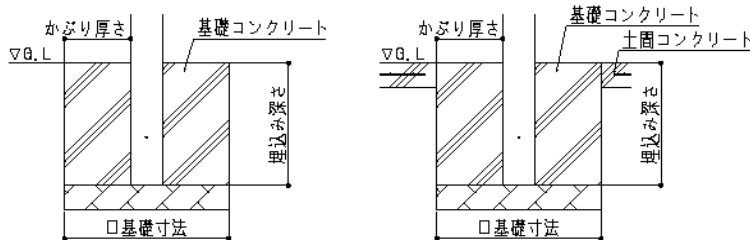
図1.基礎仕様
