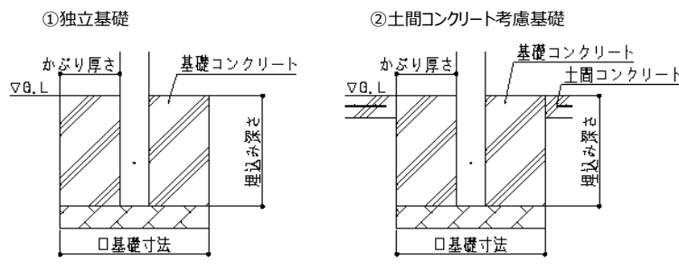
図1.基礎仕様
