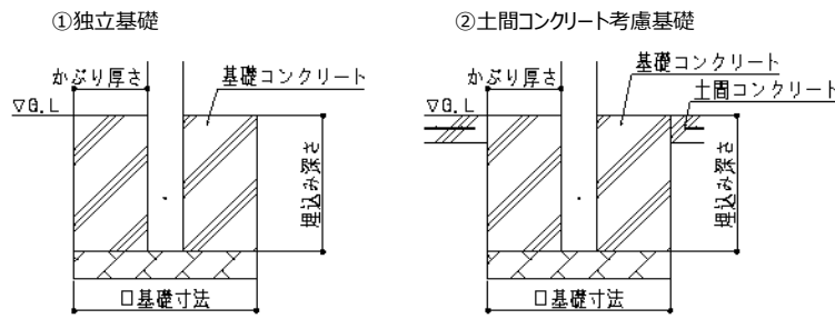
図1.基礎仕様
