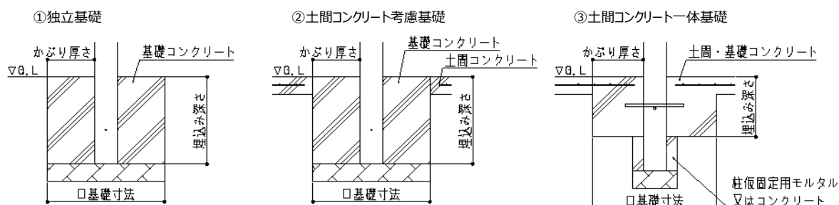
図1.基礎仕様
