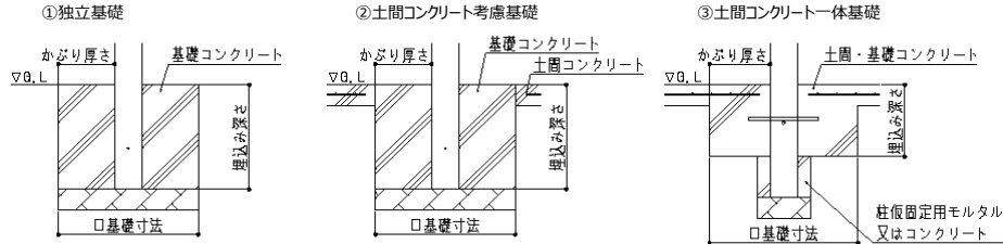
図1.基礎仕様
