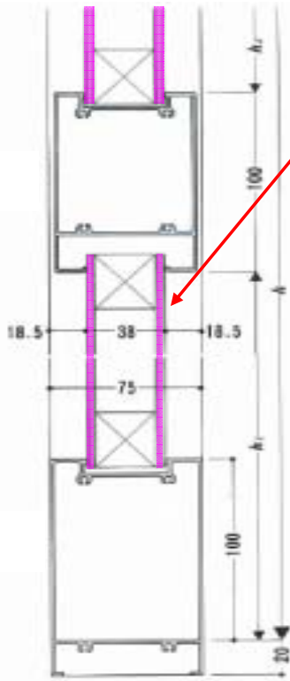
縦断面図
