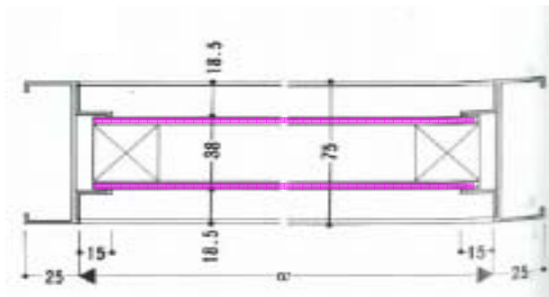
横断面図
