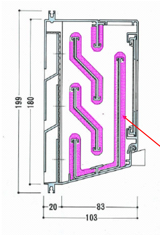
縦断面図
