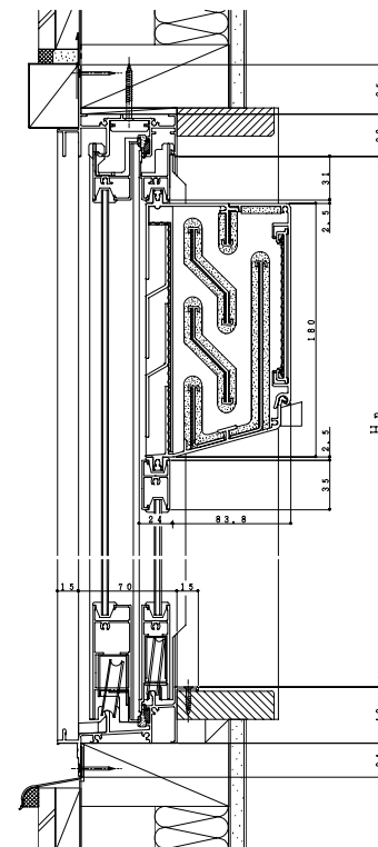
縦断面図 (取付時)
