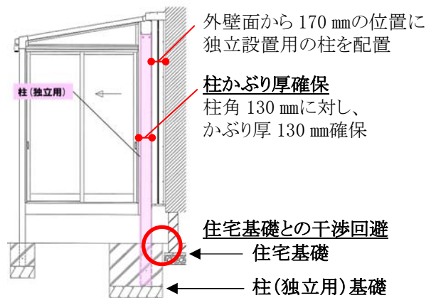
独自のフレーム構造 (日本特許出願中)
