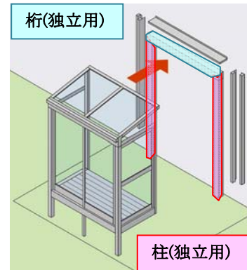
独自のフレーム構造 (日本特許出願中)
