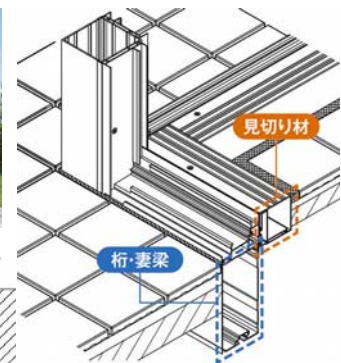
新設土間の場合の納まり
