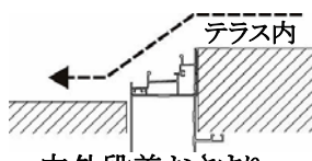
新設土間の場合の納まり
