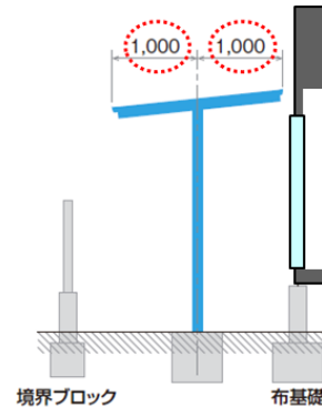
設置イメージ: 「レセパ」Tタイプ
