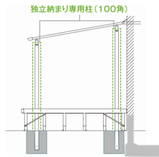
New 「サザンテラス」独立納まり (左)施工例 (右)断面図の例
