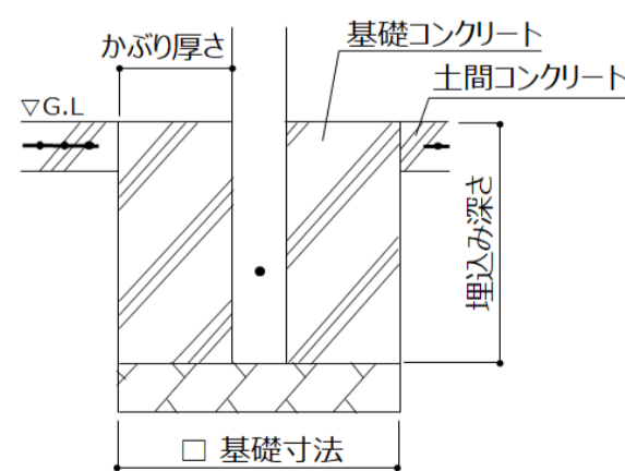
②土間コンクリート考慮基礎
