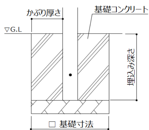
①独立基礎
