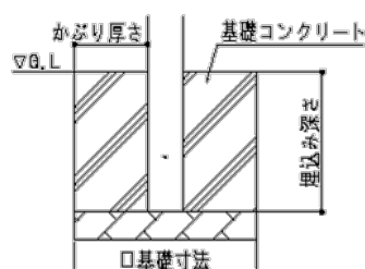
①独立基礎
