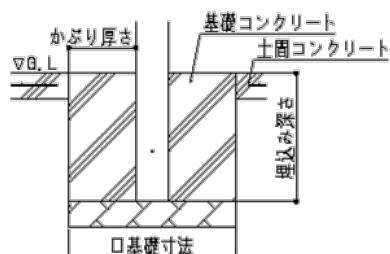
②土間コンクリート考慮基礎
