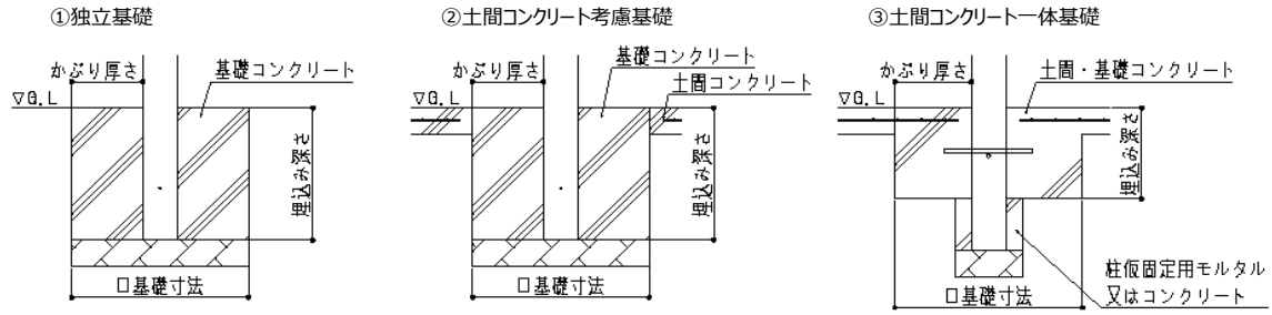
図1.基礎仕様
