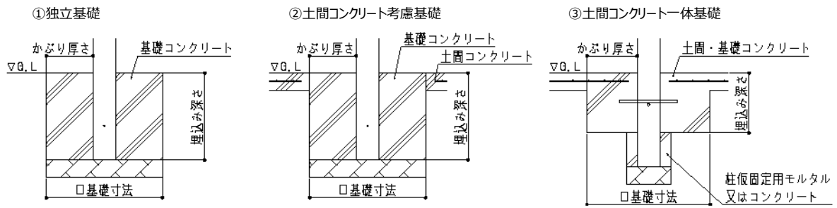
図1.基礎仕様
